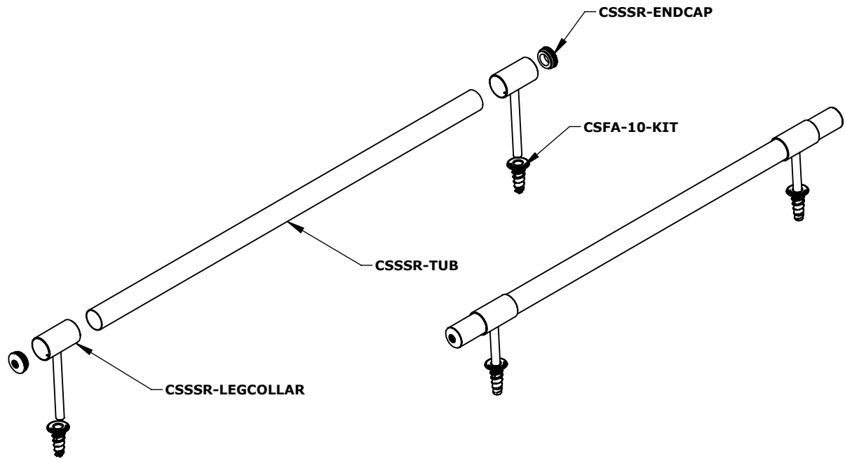
ISOMETRIC VIEW SCALE: 1:8
